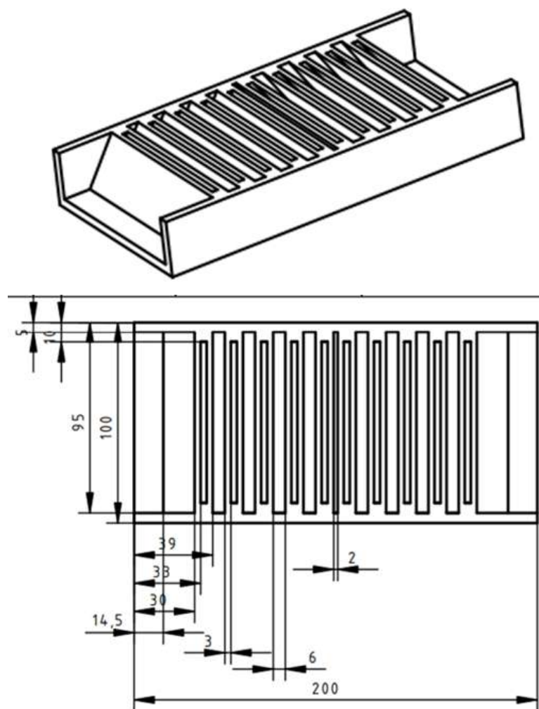
Рис. 5-6. Платформа вид снизу
