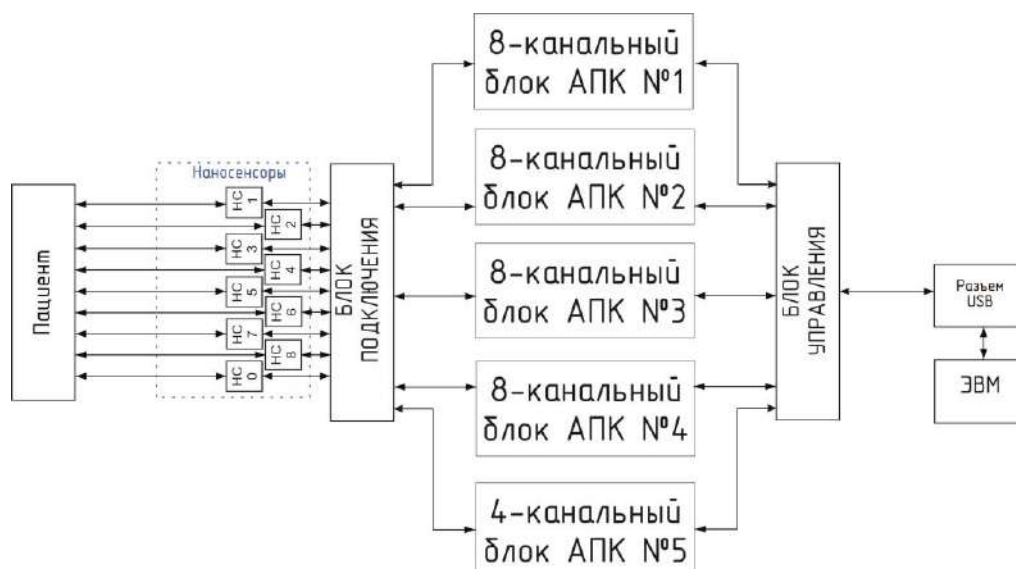
Рис. 1. Структурная схема 36-канального АПК
