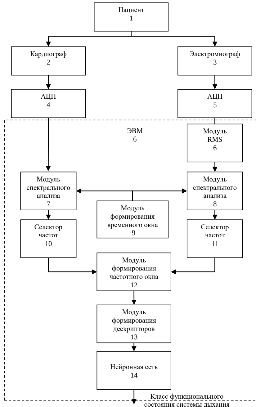
Рис. 1. Структурная схема нейросетевого классификатора медицинского риска системы дыхания
