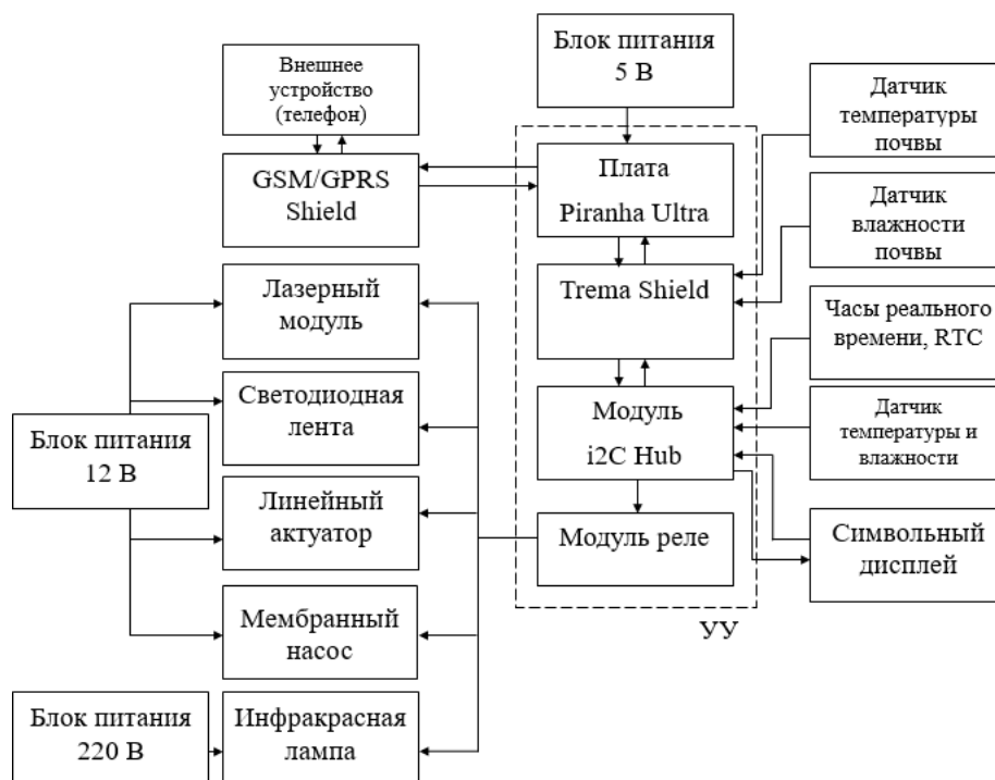
Рис. 2. Функциональная схема биотехнической системы
