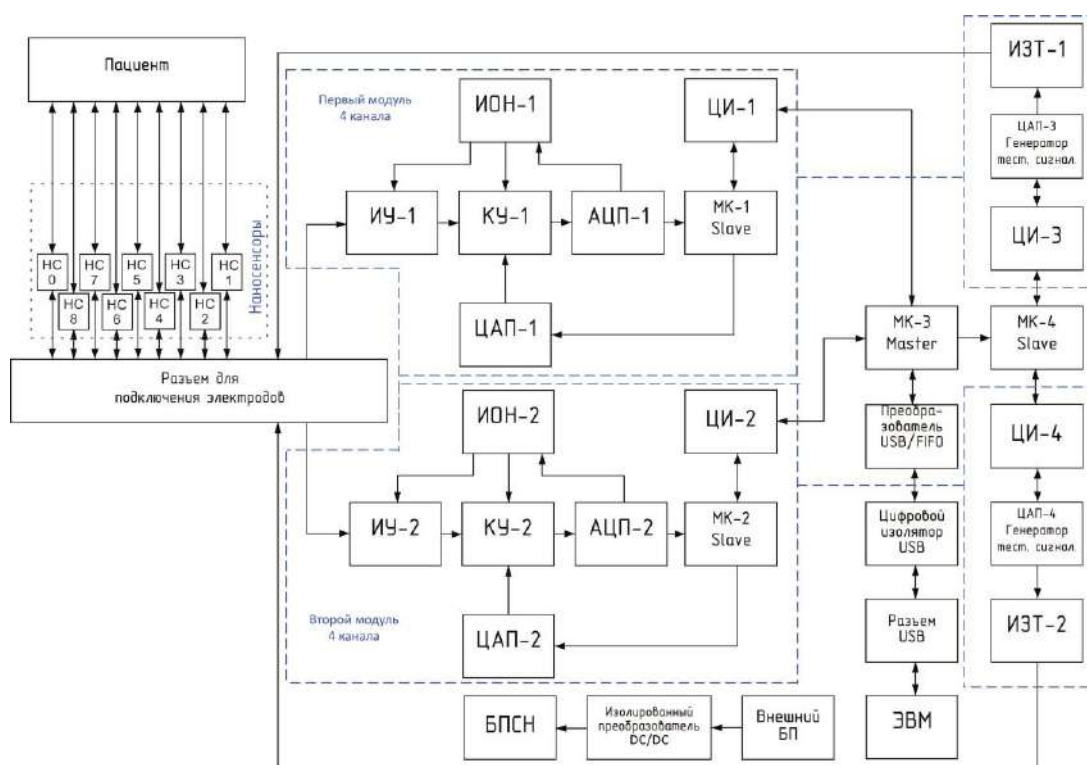
Рис. 2. Структурная схема 8-канального блока обработки ЭКГ сигналов
