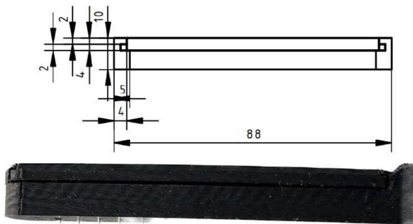
Рис 9–10. Картридж вид сбоку
