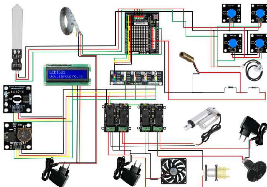
Рис. 3. Схема подключения
