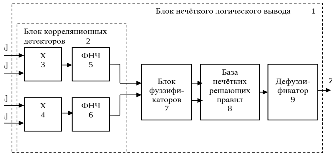
Рис. 1. Структурная схема блока нечеткого логического вывода
