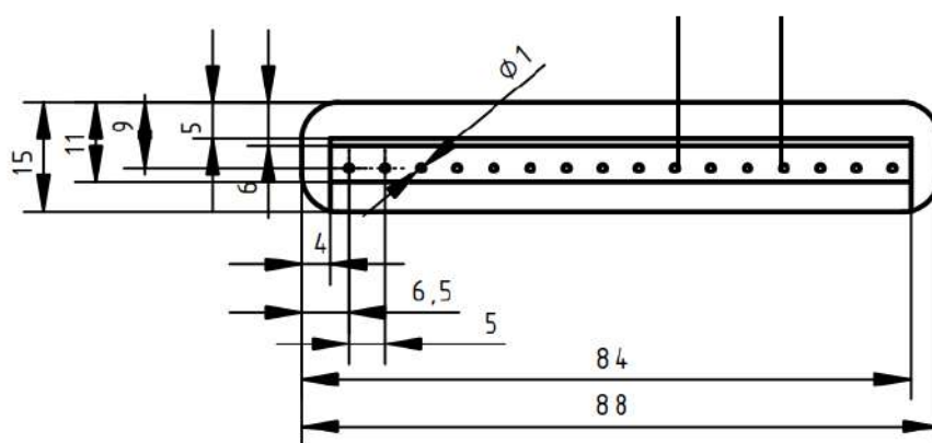
Рис. 11. Картридж вид сверху
