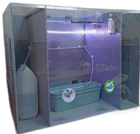
Рис. 1. Внешний вид биотехнической системы для выращивания растений
