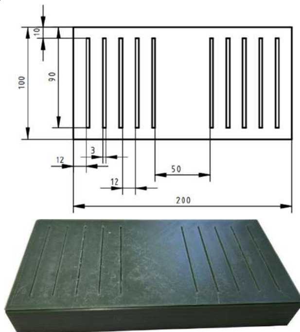
Рис. 1–2. Платформа вид сверху
